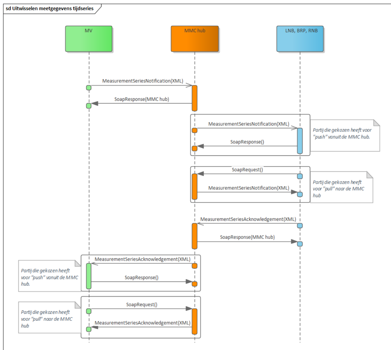
Figuur 2 Het sequence diagram voor uitwisselen meetgegevens tijdseries tussen MV en LNB, BRP en RNB via de MMC-hub
