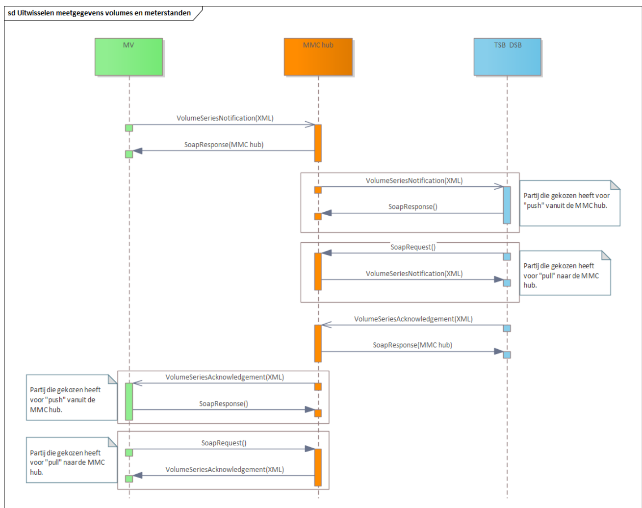
Figuur 2 Het sequence diagram voor uitwisselen volumes en meterstanden tussen MV en DSB en TSB via de MMC-hub
