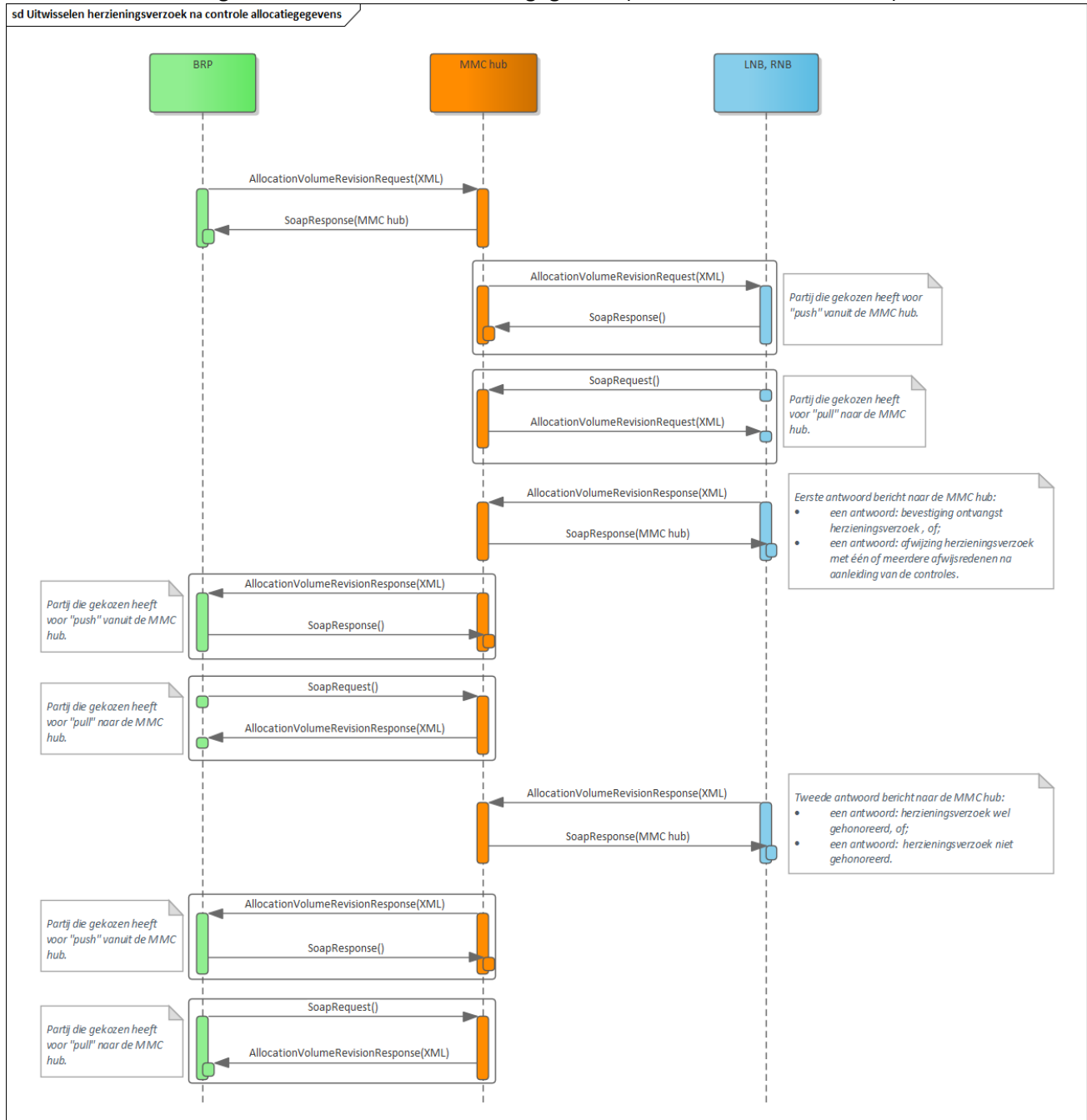
Figuur 3 Het sequence diagram voor uitwisselen van herzieningsverzoeken na controle allocatiegegevens tussen BRP en de LNB of RNB via de MMC-hub
