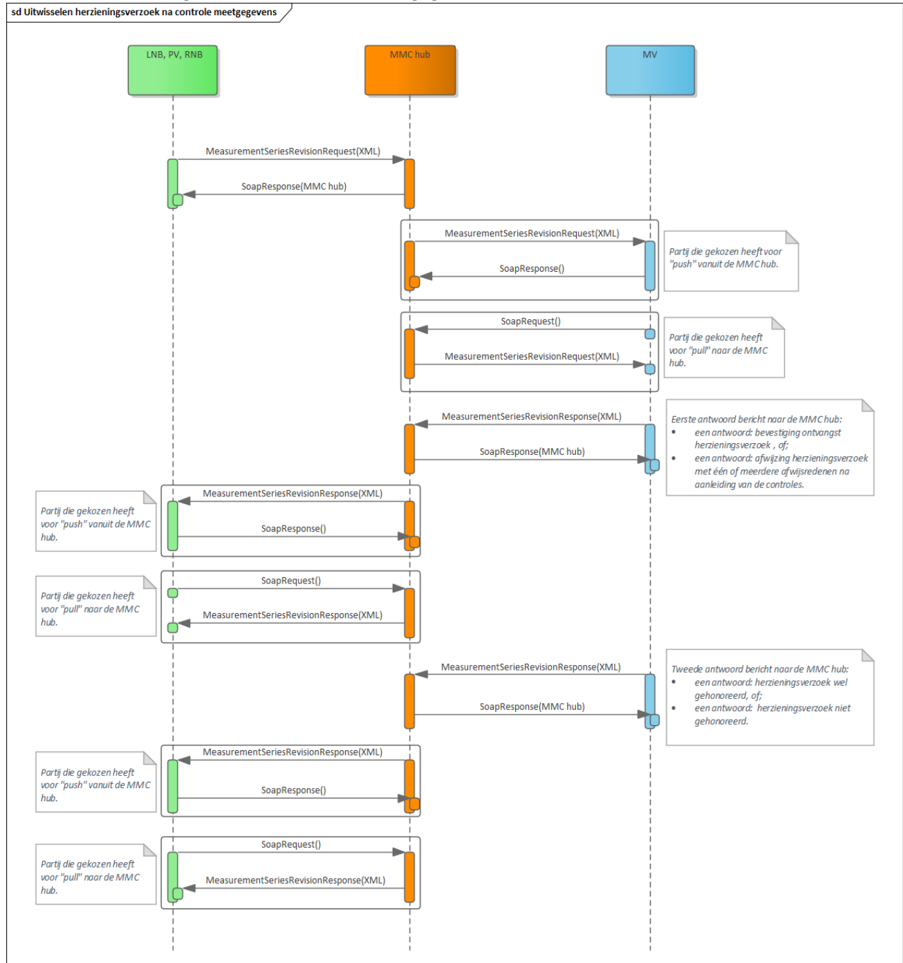
Figuur 2 Het sequence diagram voor uitwisselen van herzieningsverzoeken na controle meetgegevens tussen LNB, PV of RNB en de MV via de MMC-hub
