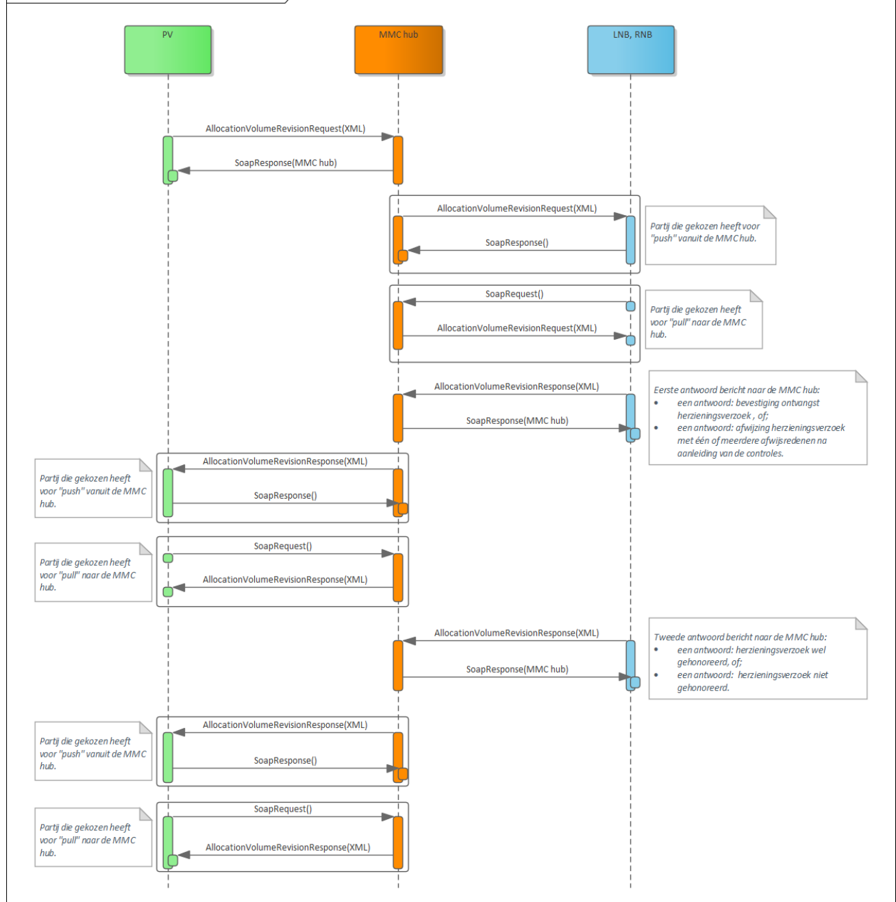
Figuur 3 Het sequence diagram voor uitwisselen van herzieningsverzoeken na controle allocatiegegevens tussen PV en de LNB of RNB via de MMC-hub
