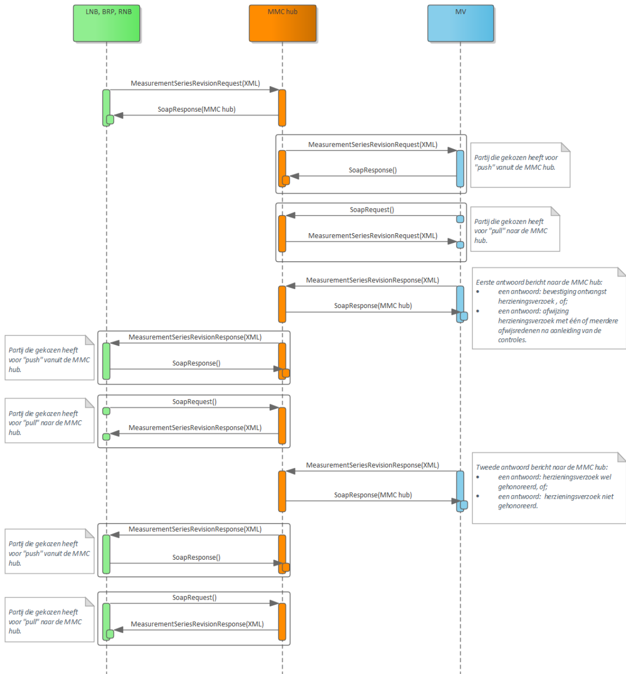
Figuur 2 Het sequence diagram voor uitwisselen van herzieningsverzoeken na controle meetgegevens tussen LNB, BRP of RNB en de MV via de MMC-hub
