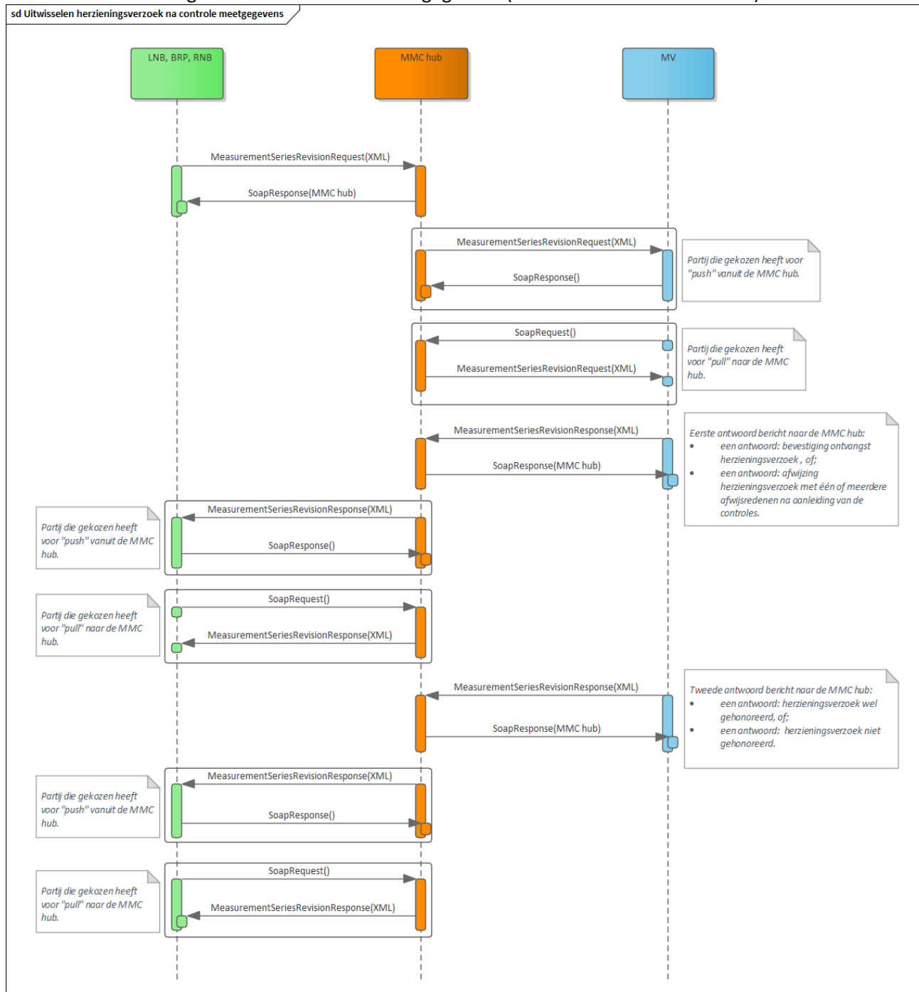
Figuur 2 Het sequence diagram voor uitwisselen van herzieningsverzoeken na controle meetgegevens tussen LNB, BRP of RNB en de MV via de MMC-hub
