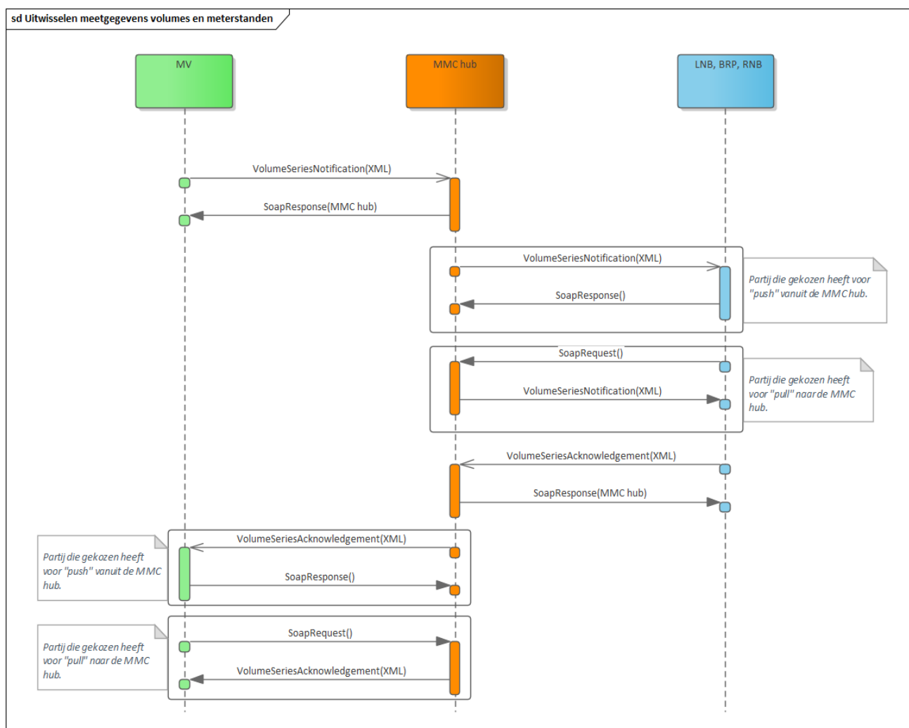
Figuur 2 Het sequence diagram voor uitwisselen volumes en meterstanden tussen MV en LNB, BRP en RNB via de MMC-hub
