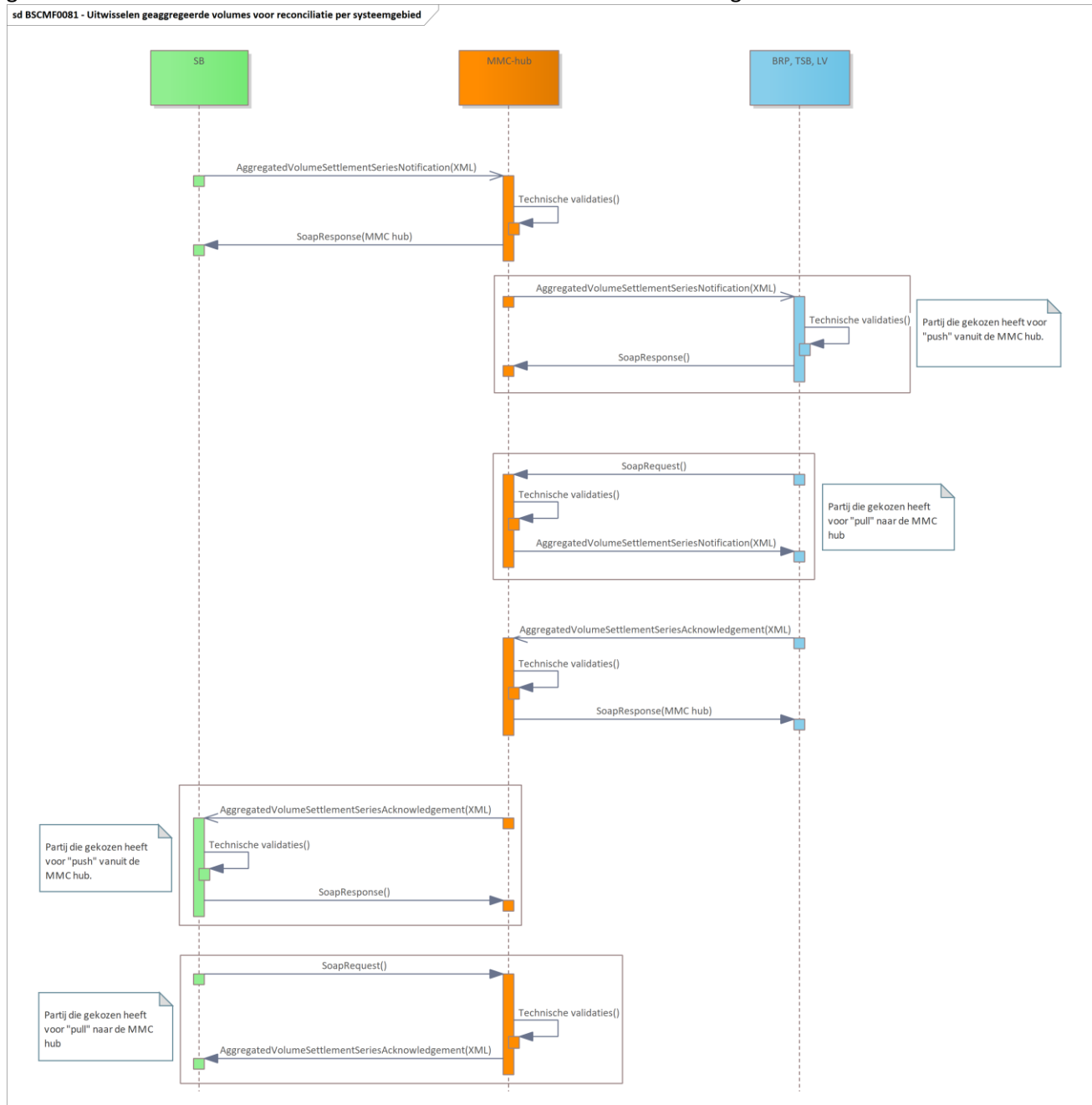
Figuur 2 Het sequence diagram voor uitwisselen volumes voor reconciliatie tussen SB en BRP, TSB en LV via de MMC-hub
