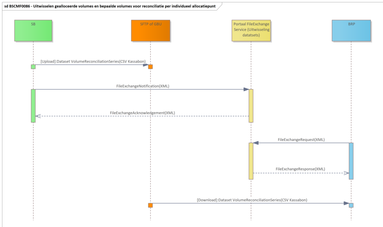
Figuur 7 Het sequence diagram voor uitwisselen volumes voor reconciliatie tussen SB en BRP
