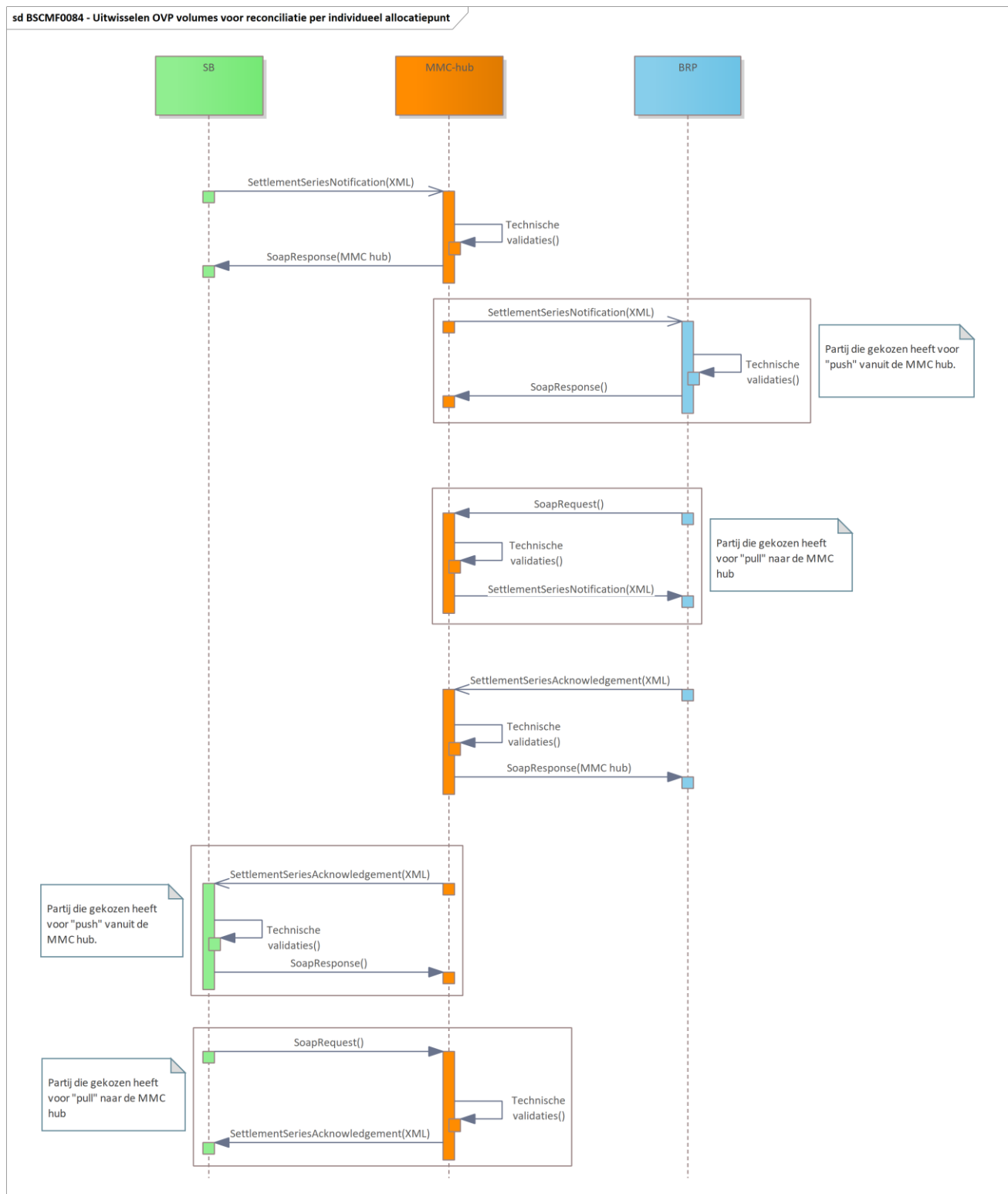
Figuur 5 Het sequence diagram voor uitwisselen volumes voor reconciliatie tussen SB en BRP via de MMC-hub
