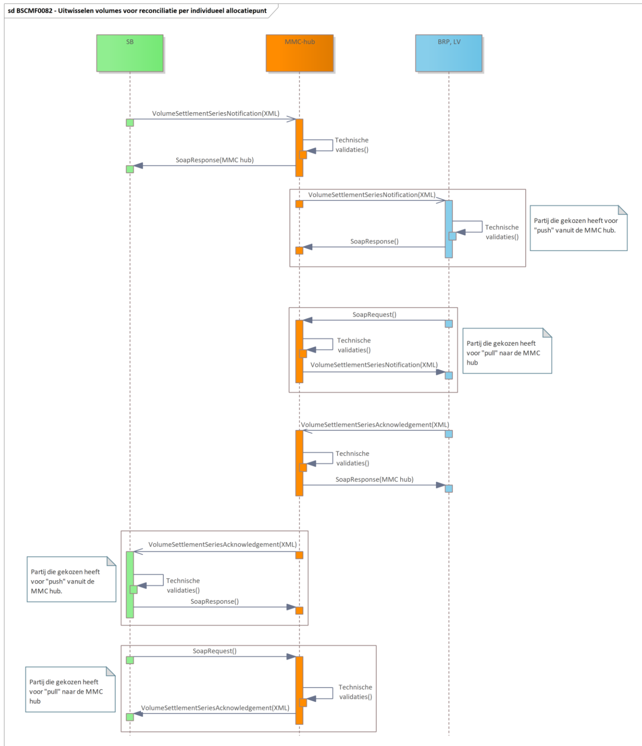
Figuur 3 Het sequence diagram voor uitwisselen volumes voor reconciliatie tussen SB en BRP en LV via de MMC-hub
