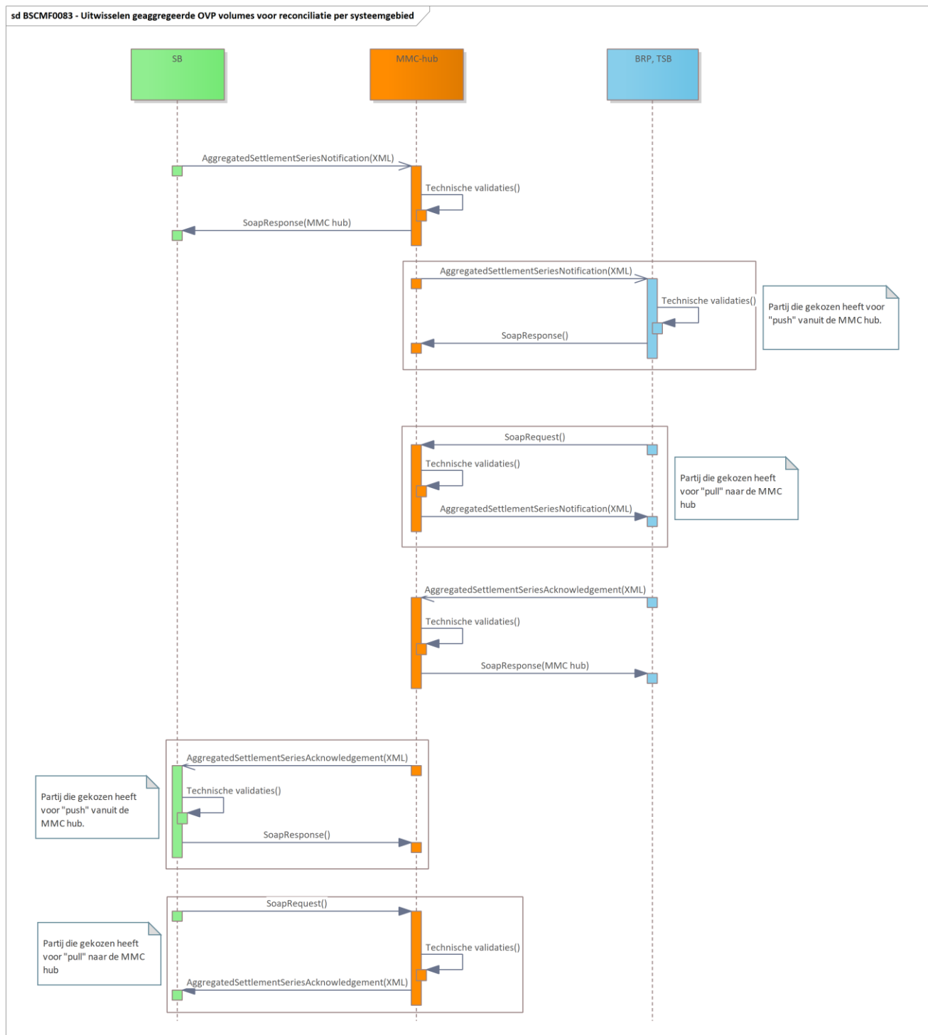
Figuur 4 Het sequence diagram voor uitwisselen volumes voor reconciliatie tussen SB en BRP en TSB via de MMC-hub
