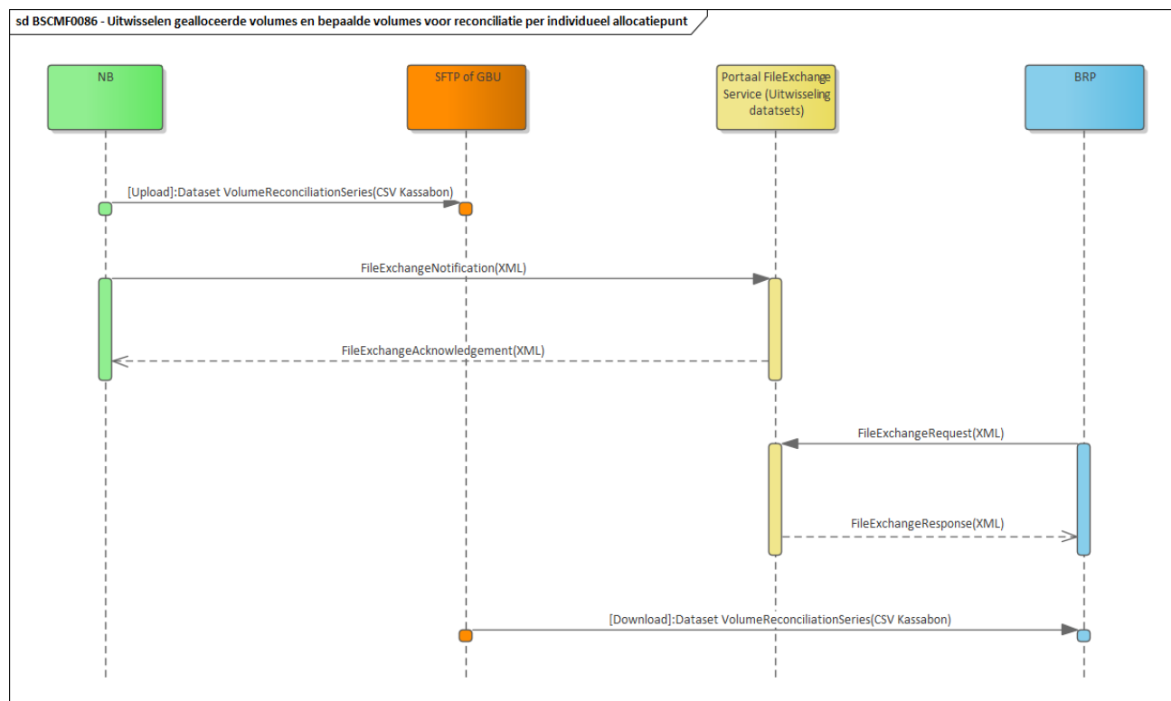
Figuur 6 Het sequence diagram voor uitwisselen volumes voor reconciliatie tussen NB en BRP
